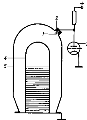
Рис. 5. Схема регулирования электростатического генератора с коронирующим электродом: 1 — коронирующие острия; 2 — изолятор; 3 — регулирующий триод; 4 — высоковольтный электрод генератора; 5 — сосуд высокого давления.
